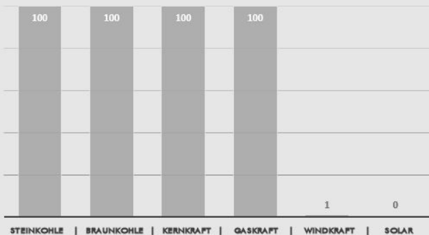
Grundlastfähige Leistung [%]
